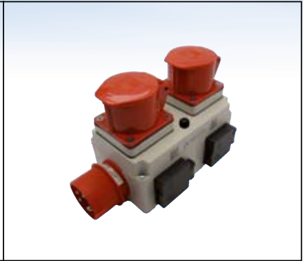
Einschaltfrietomat 1 M zum Betreiben von 1 drehstrom- bzw. 1 wechselstromgetriebenen Maschine sowie 1 Entstauber mit 230V oder 400V. Mit Phasenwender (erweiterbar bis 8 Maschinen).
