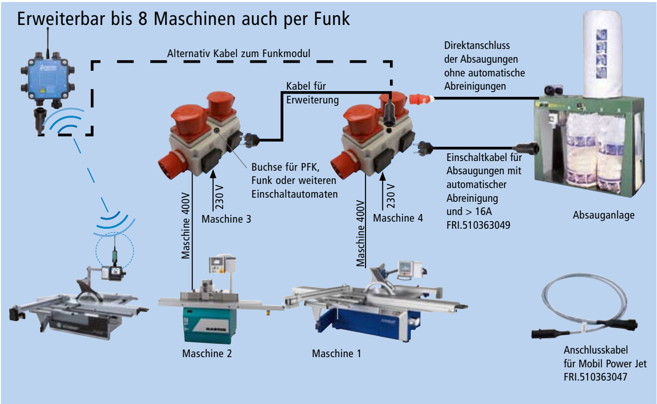
Einschaltfrietomat 1 M zum Betreiben von 1 drehstrom- bzw. 1 wechselstromgetriebenen Maschine sowie 1 Entstauber mit 230V oder 400V. Mit Phasenwender (erweiterbar bis 8 Maschinen).
